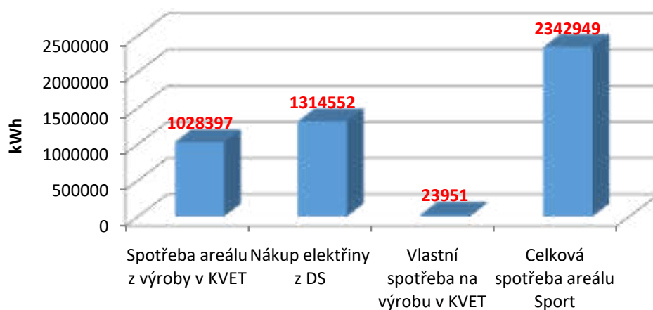
Celková spotřeba kWh Sportarálu 2018
