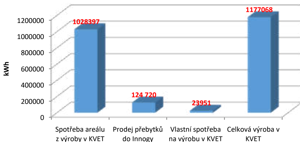
Kogenerační jednotka 2018 spotřeba, výroba a prodej
